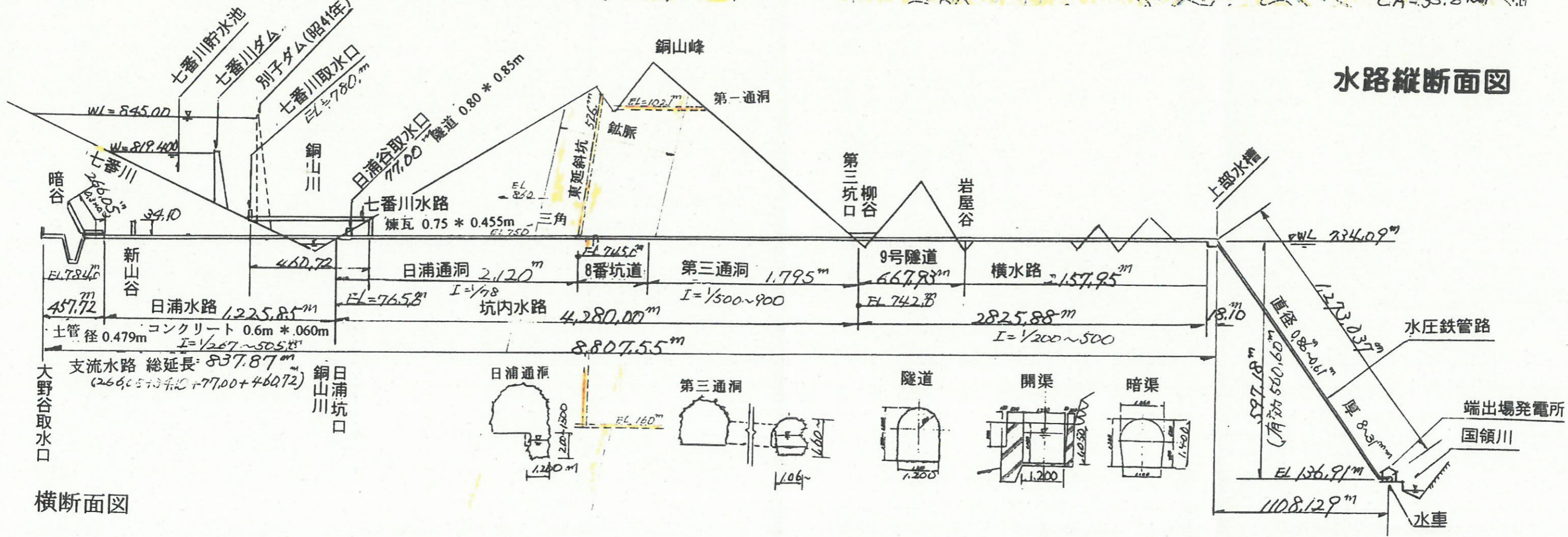
端出場水力発電所概要説明図
